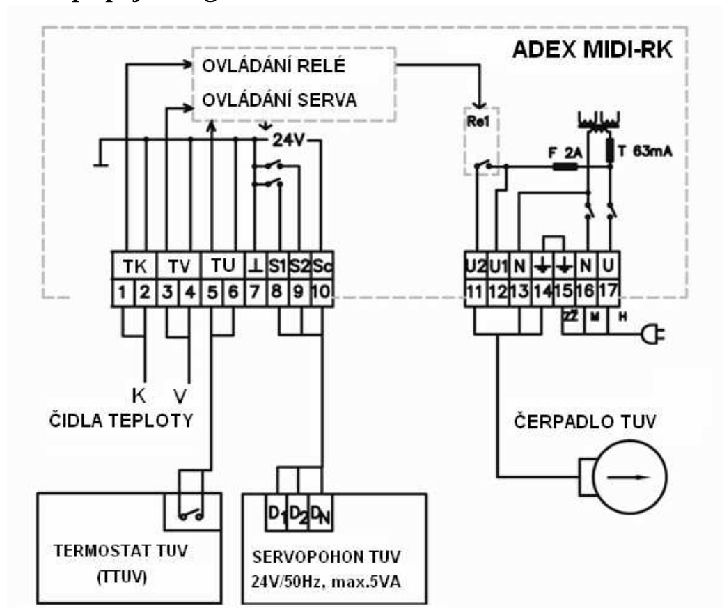
Obr. 11 Elektrické připojení regulátoru
