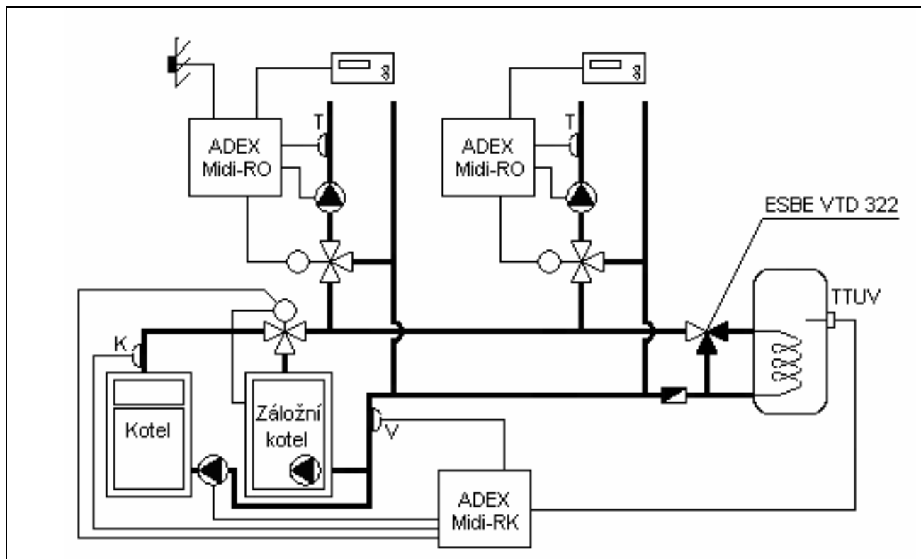
Obr. 6 Topný systém se záložním kotlem
