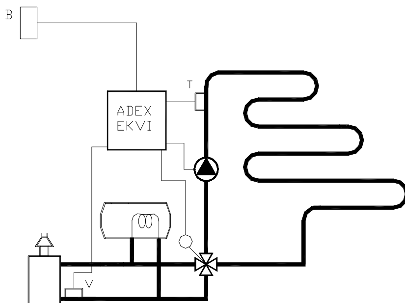
Obr.5 Příklad použití regulátoru ADEX Ekvi 2.1 pro podlahové vytápění (osazeno přídatné čidlo V pro ochranu kotle proti nízkoteplotní korozi)
