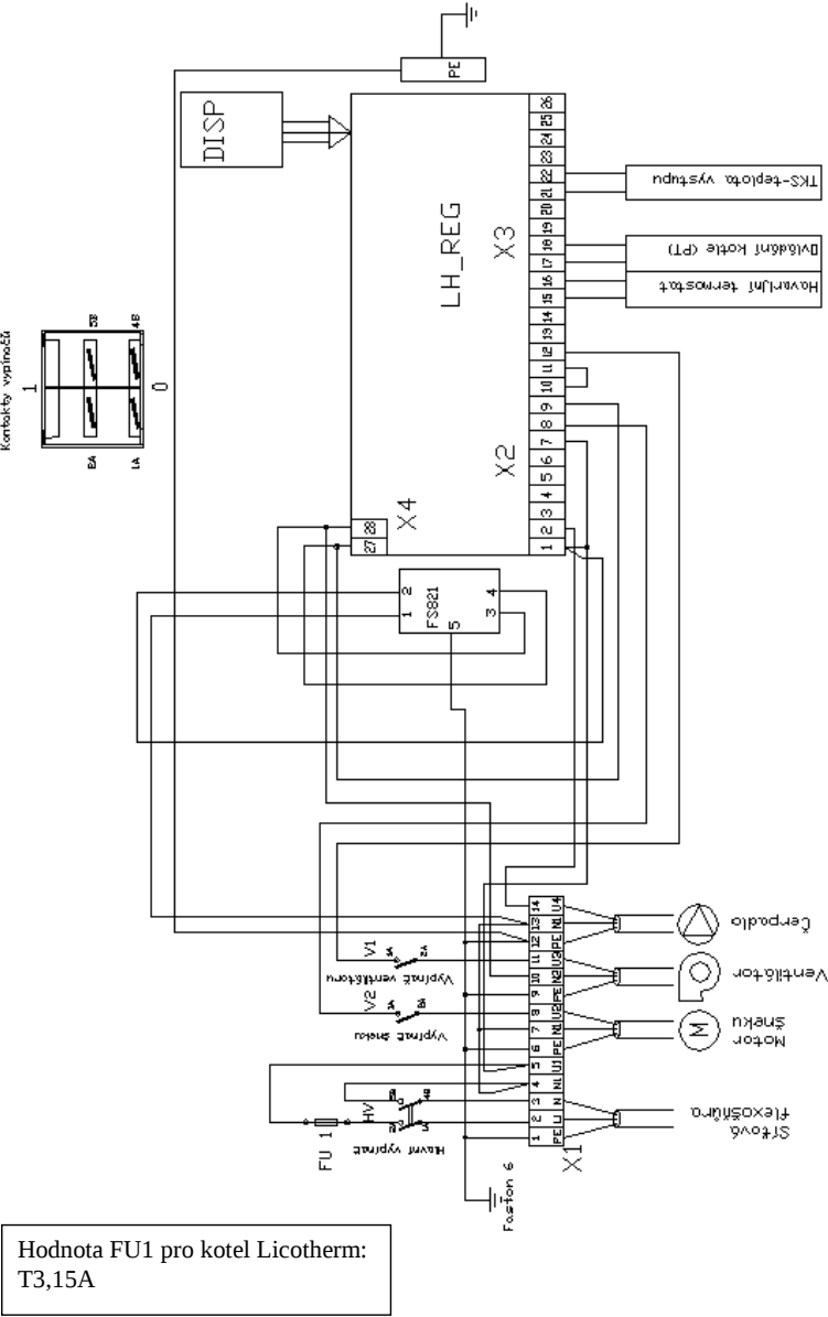
Obr. 2 Svorkové schéma regulátoru ADEX LH_REG/Licotherm
