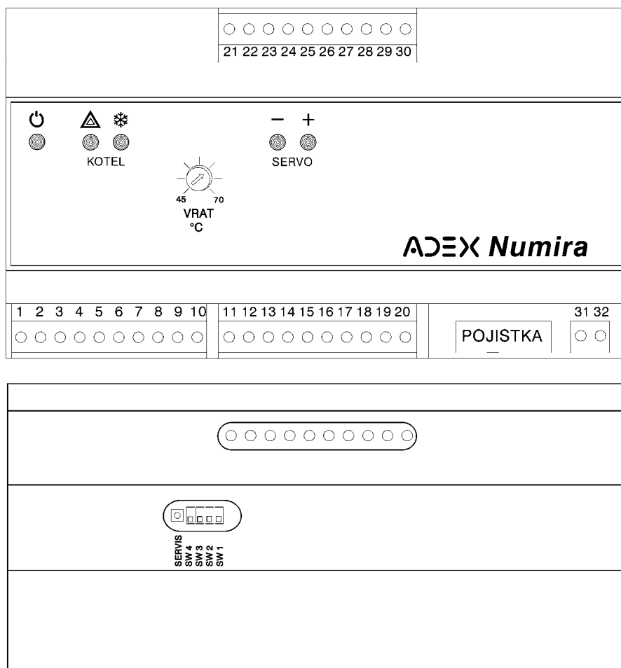
Obr. 7 Hlavní prvky regulátoru
