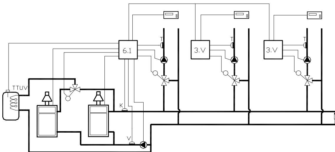
Obr. 6b Zapojení s regulátory ADEX Numira 3.V - pro ohřev TUV se přepíná první kotel Upozornění: K ovládání přepínacího ventilu TUV nutno použít 2-bodový servopohon 230 V.
