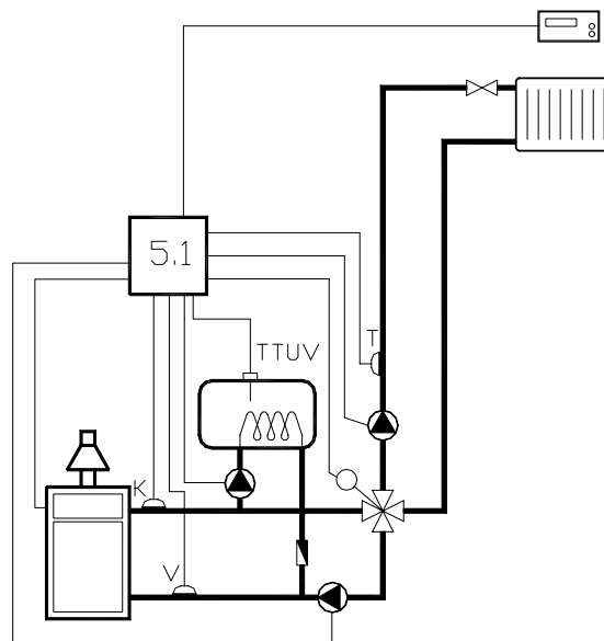
Obr. 4 Typické zapojení regulátoru ADEX Numira 5.1
