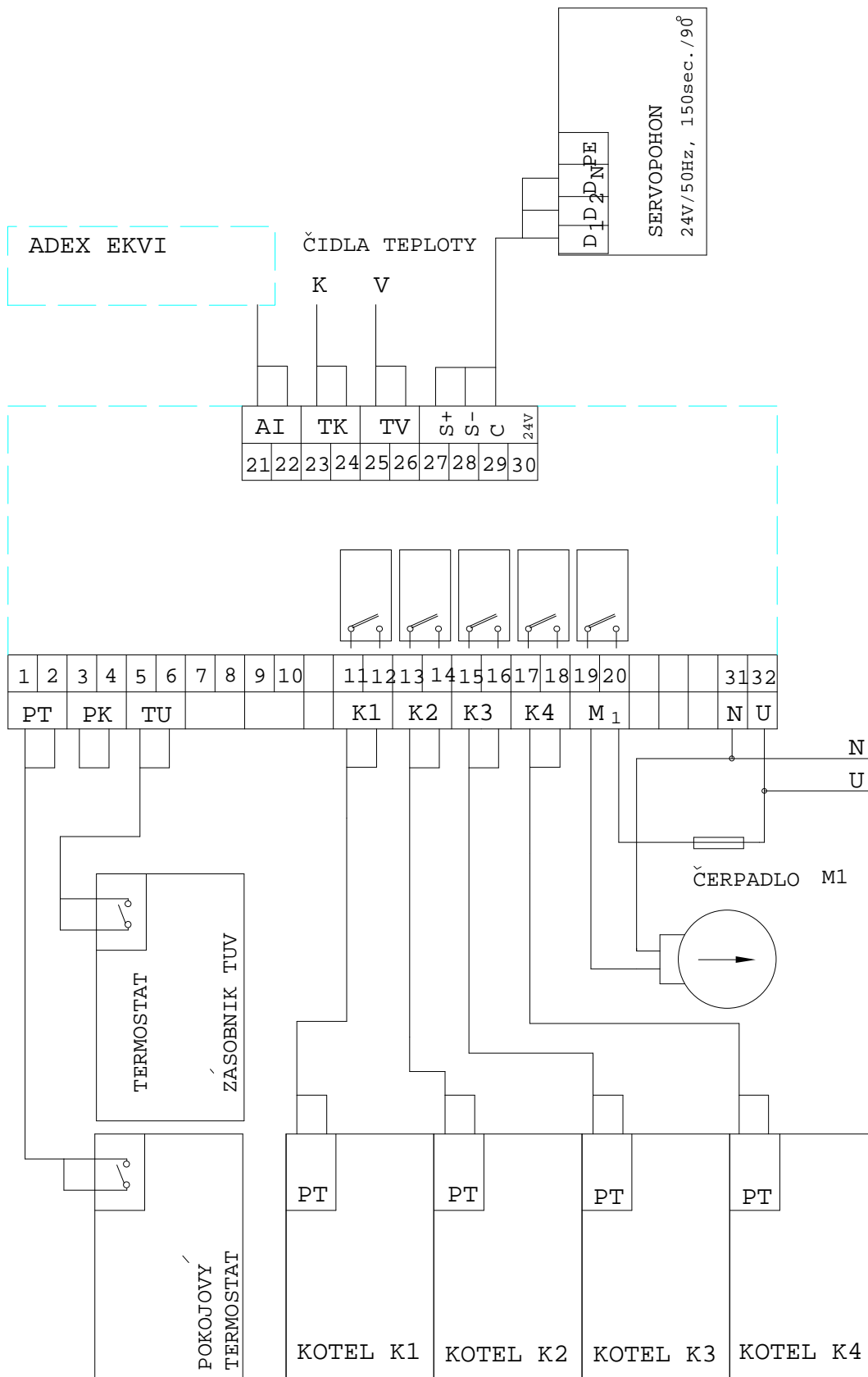
Obr.4 Zapojení připojovací svorkovnice regulátoru
