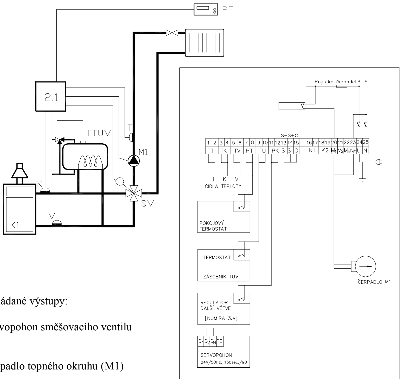
Zapojovací schéma ADEX Numira 2.1
